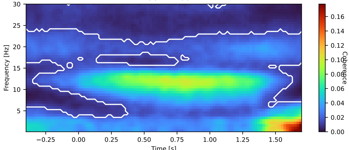
8B (3) - dPFC (7)
